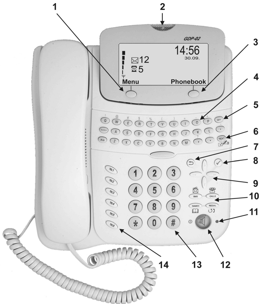
Bild 3: Ansicht des Telefons von oben
